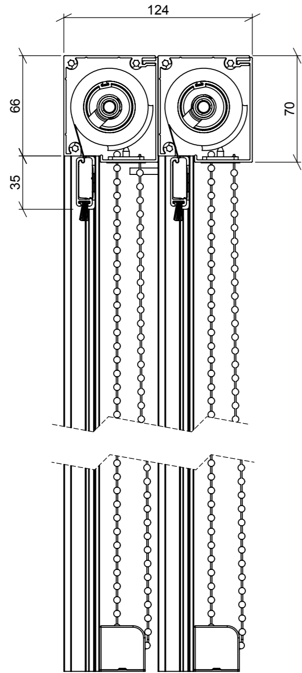
SECTION A-A
