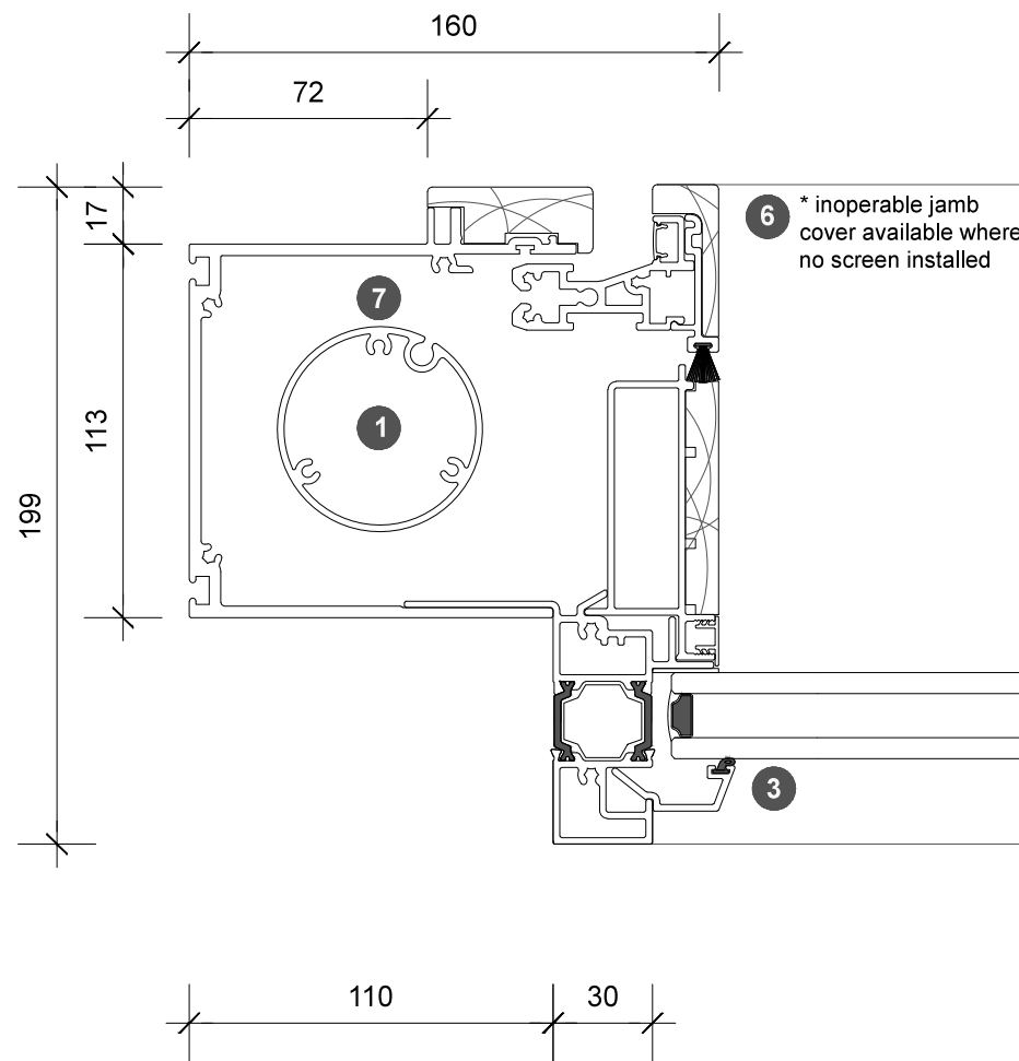
1. jamb detail
