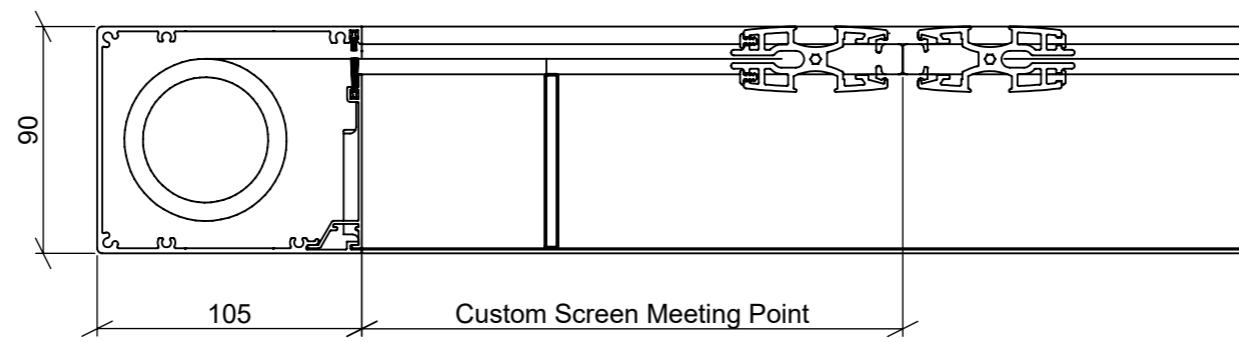
SECTION B-B SCALE 1 : 3
