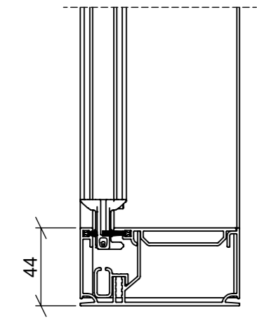
SECTION A-A SCALE 1 : 3
