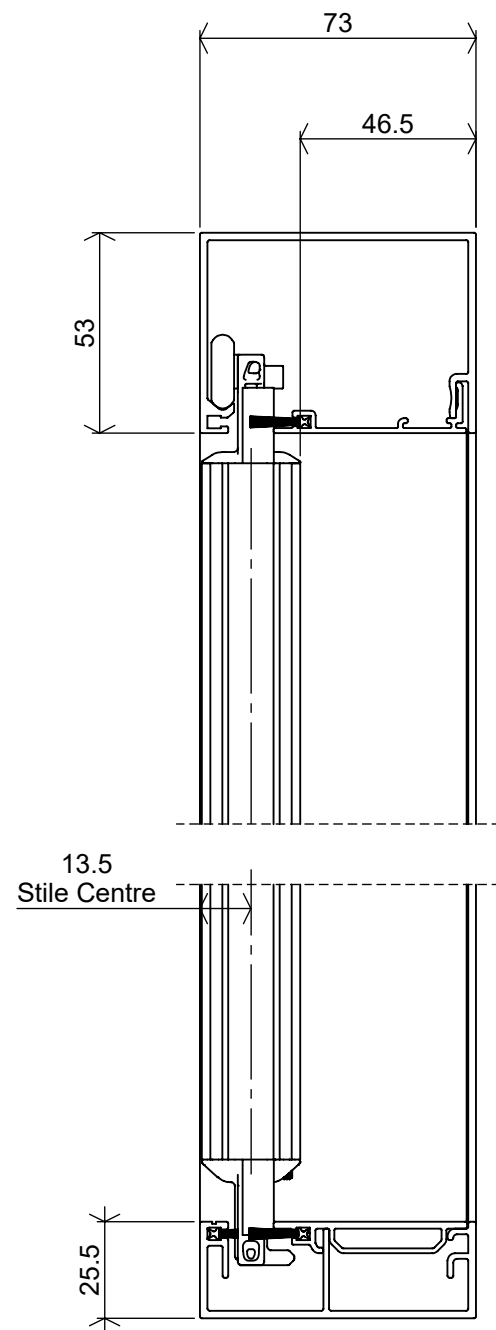
SECTION A-A
