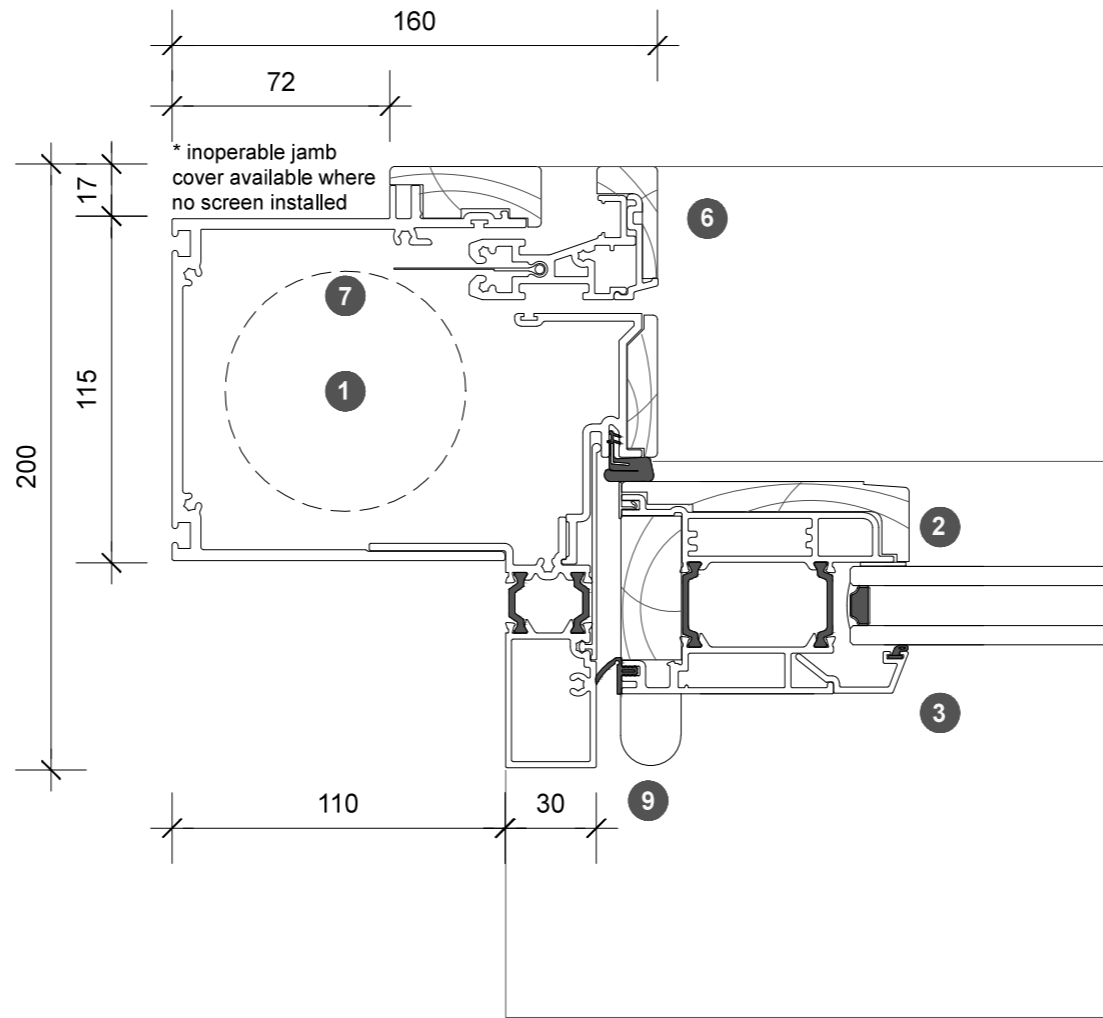
1. jamb detail
