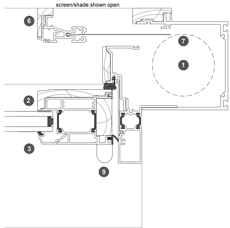
2. jamb detail
