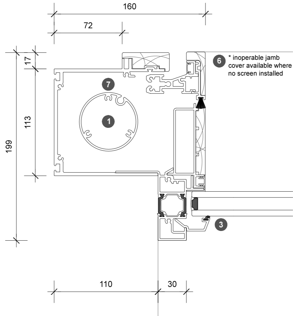
1. jamb detail
