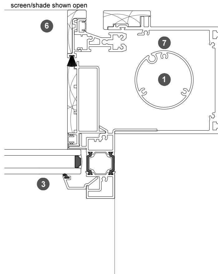
3. jamb detail
