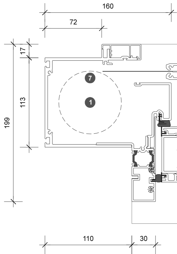
1. jamb detail
