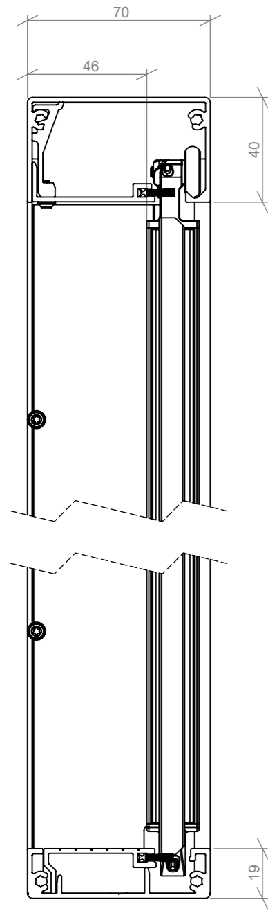
SECTION A-A
