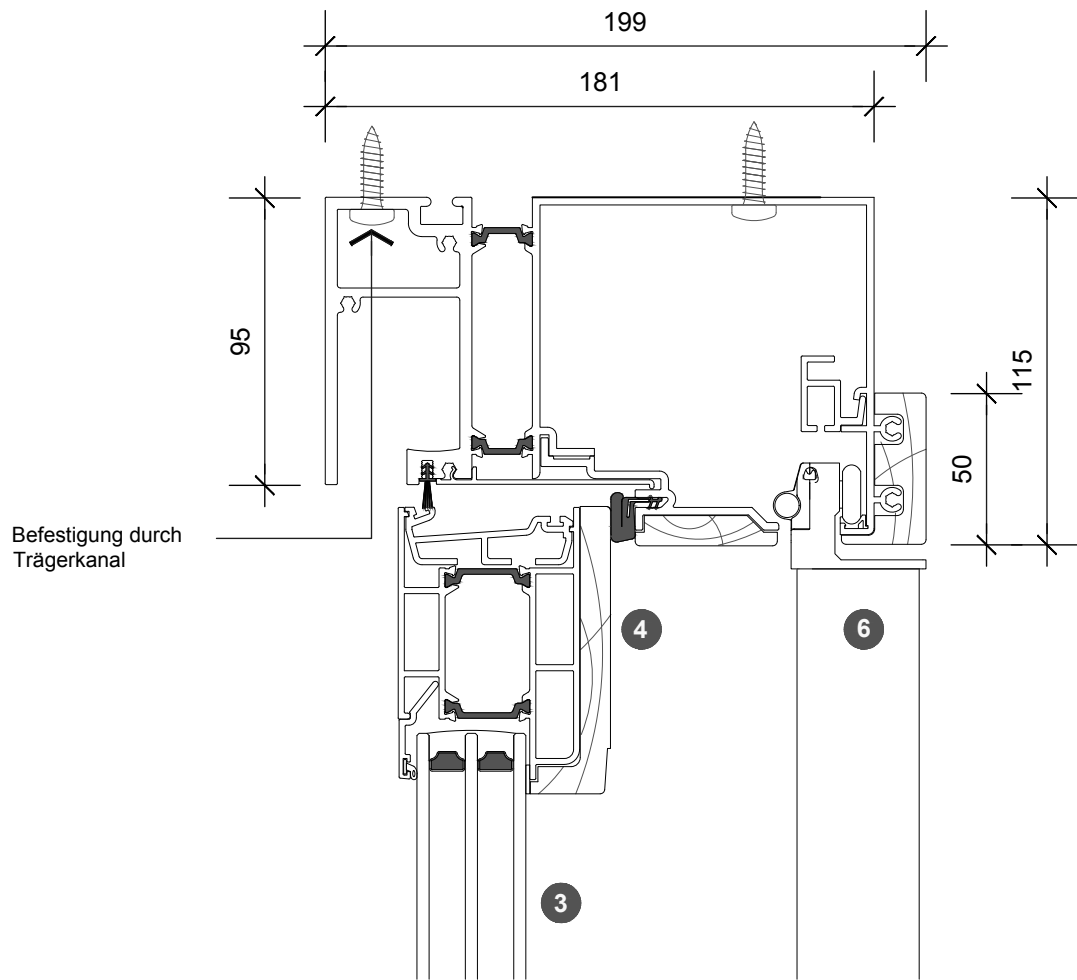
3. Kopfprofil-Detail
