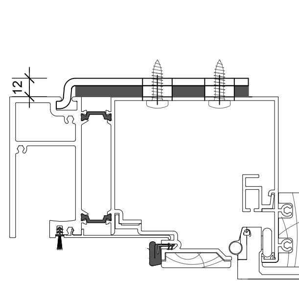
3a. Kopfprofil (mit Kopfmontageplatte)
