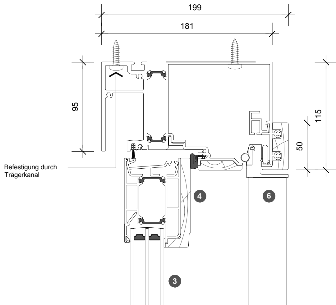
3. Kopfprofil-Detail
