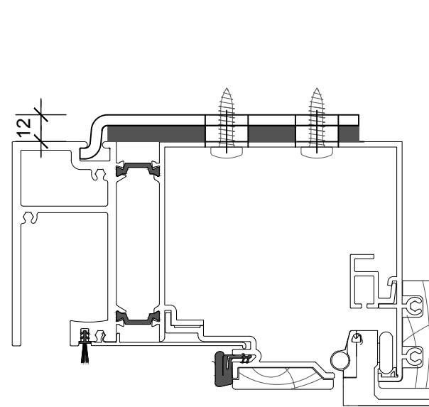
3a. Kopfprofil (mit Kopfmontageplatte)
