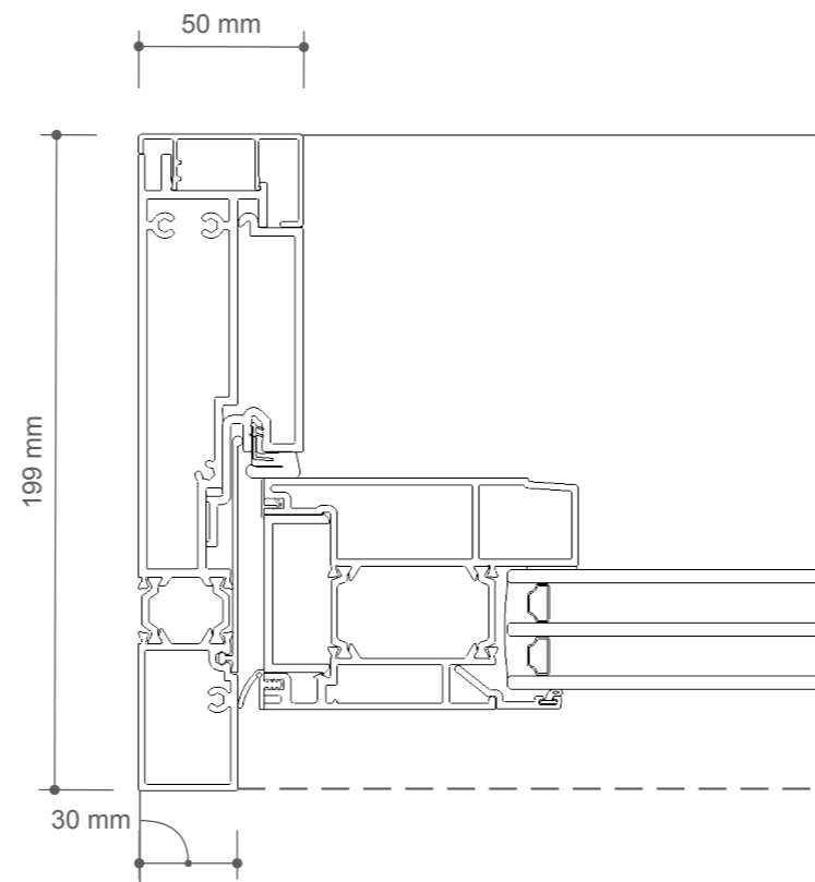
1. Jamb detail
