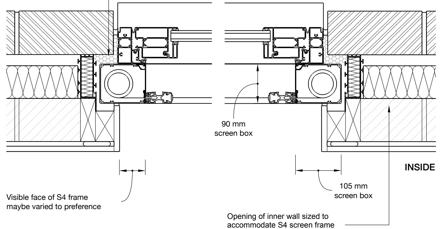
Horizontal section - Jamb
