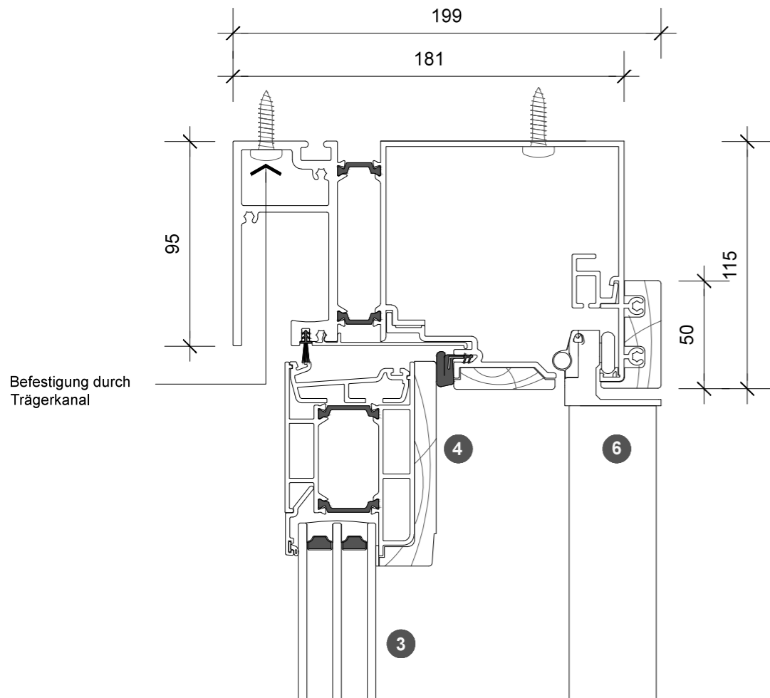
3. Kopfprofil-Detail
