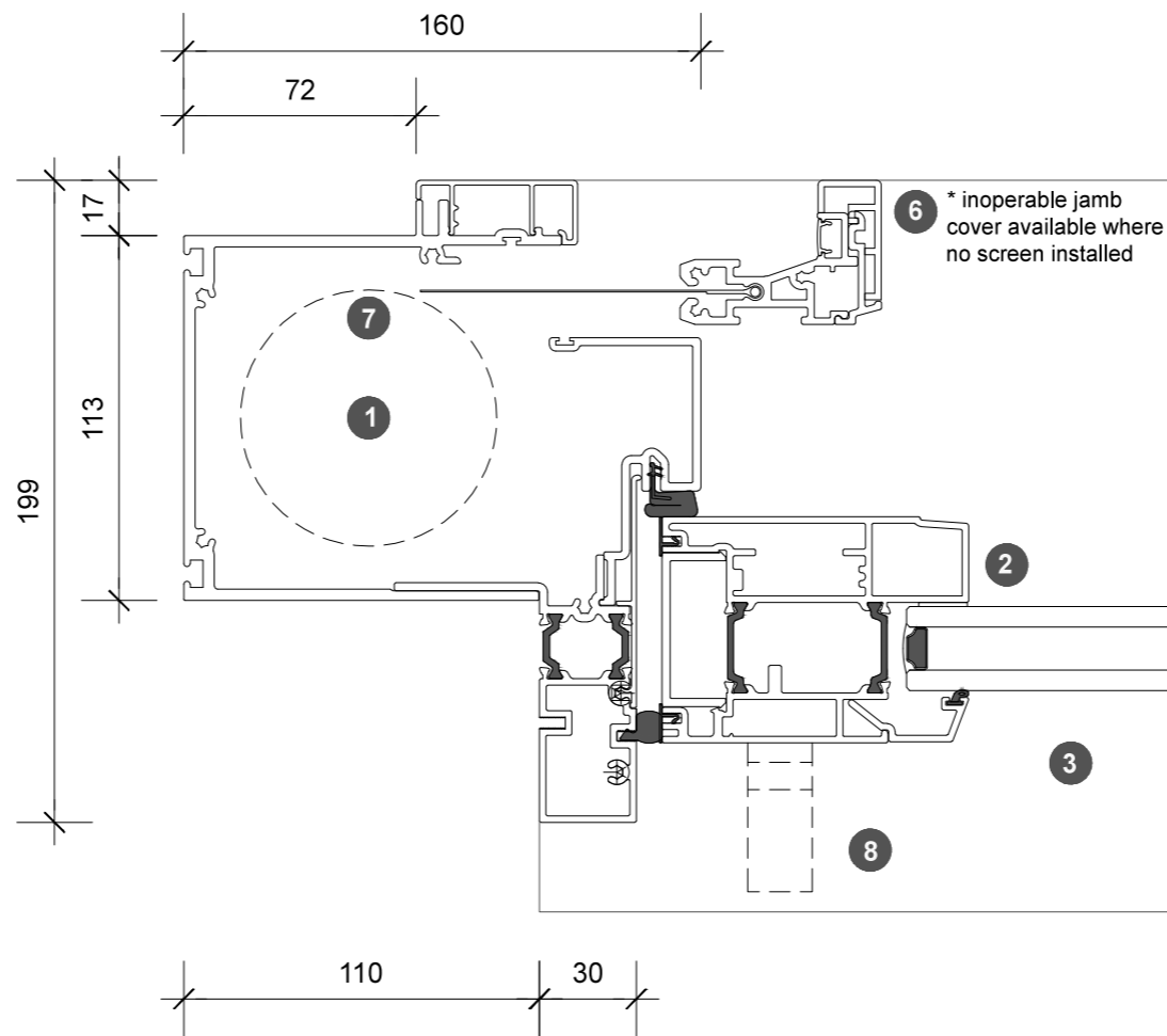
1. jamb detail
