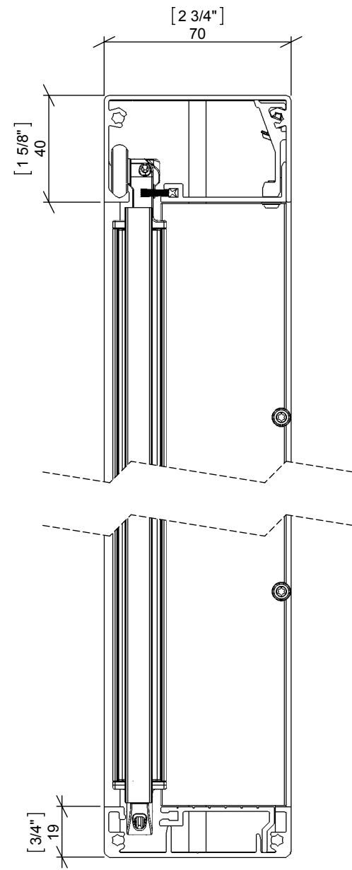
SECTION A-A
